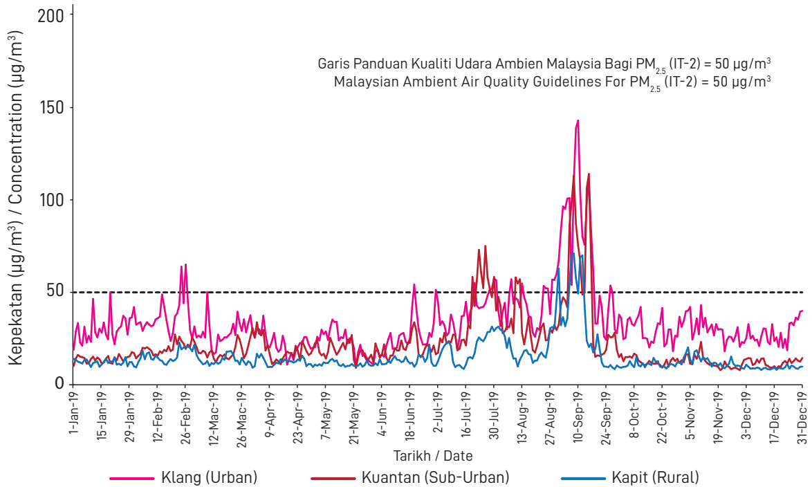
Rajah 1.1 (b) : Tren Kepekatan 24 jam bagi Habuk Halus Bersaiz 2.5 Mikron ( PM_{2.5} ), Malaysia, 2019
