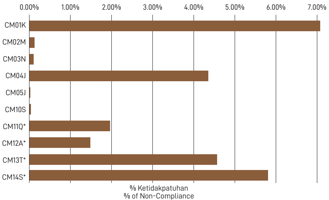
Rajah 4.6: Peratus Ketidakpatuhan Parameter Jumlah Pepejal Terampai Berdasarkan Standad Kualiti Air Marin Malaysia
