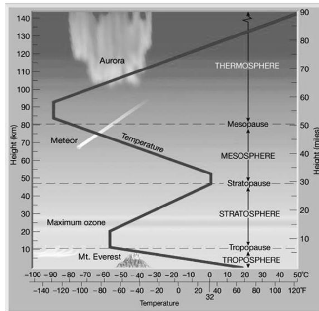
Rajah 2: Struktur Lapisan Atmosfera
