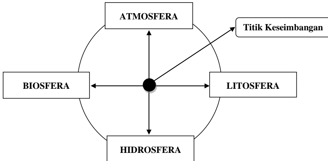
Rajah 1: Sistem Alam Sekitar Fizikal dan Perhubungannya (Sumber: Hamidi Ismail et.al, 2004)
