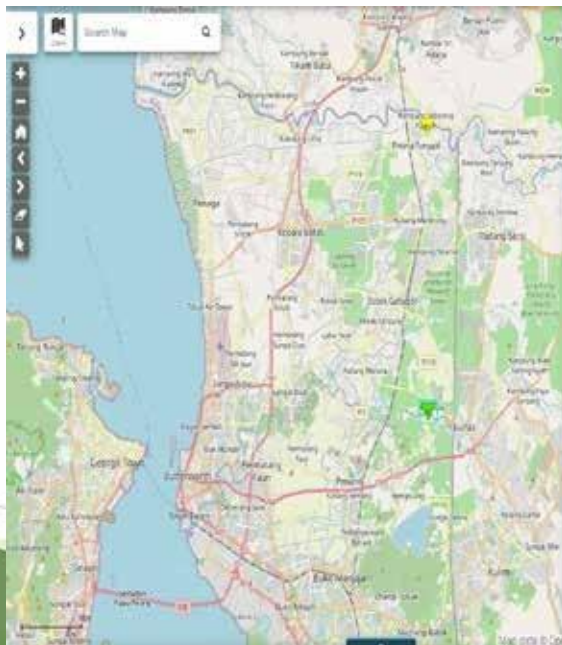
Rajah 3.11: Peta menunjukkan Stesen Pengawasan Sungai Automatik
