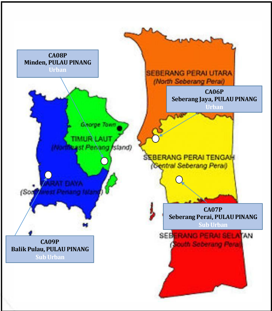
Rajah 3.6: Peta menunjukkan kedudukan stesen udara automatik Jabatan Alam Sekitar Pulau Pinang
