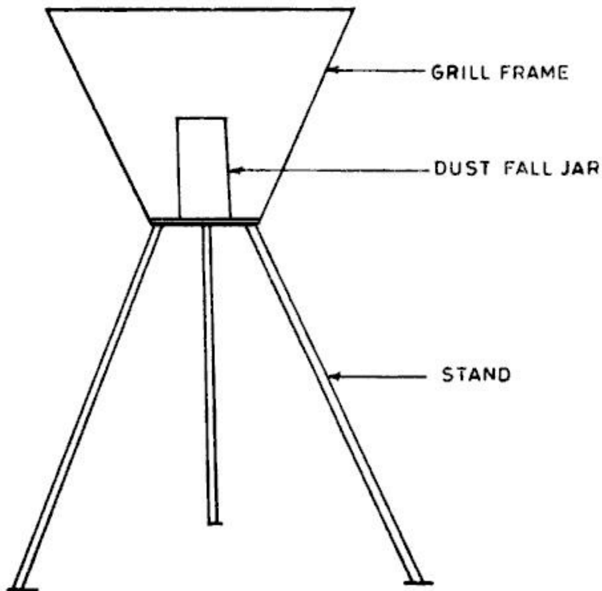
Fig. 9.2 Dust fall jar
