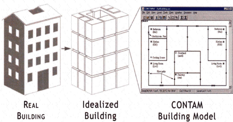
Fig. 10.11 CONTAM 2.4 program.
