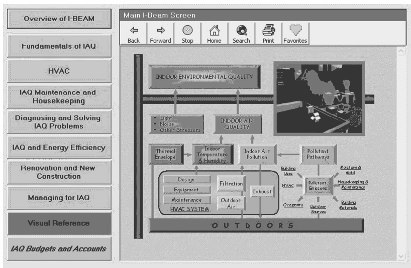
Fig. 10.12 I-BEAM program.
