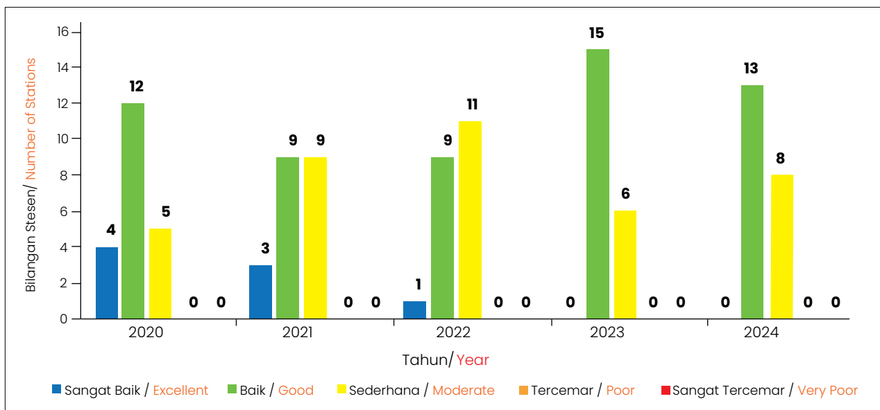
Rajah 3.3: Trend Indeks Kualiti Air Tanah bagi Tapak Perindustrian, 2020 - 2024
